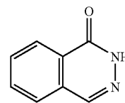
phthalazinone
