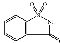
saccharin
