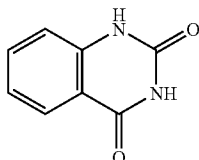
quinazolidine-2,4-dione
