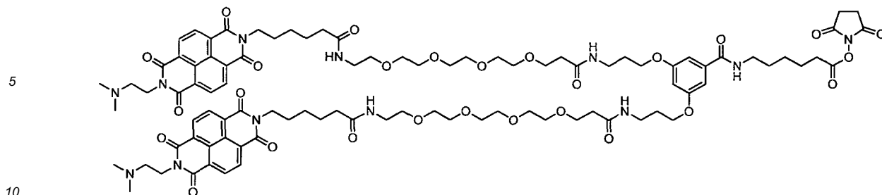
Bis-NDI-C6
