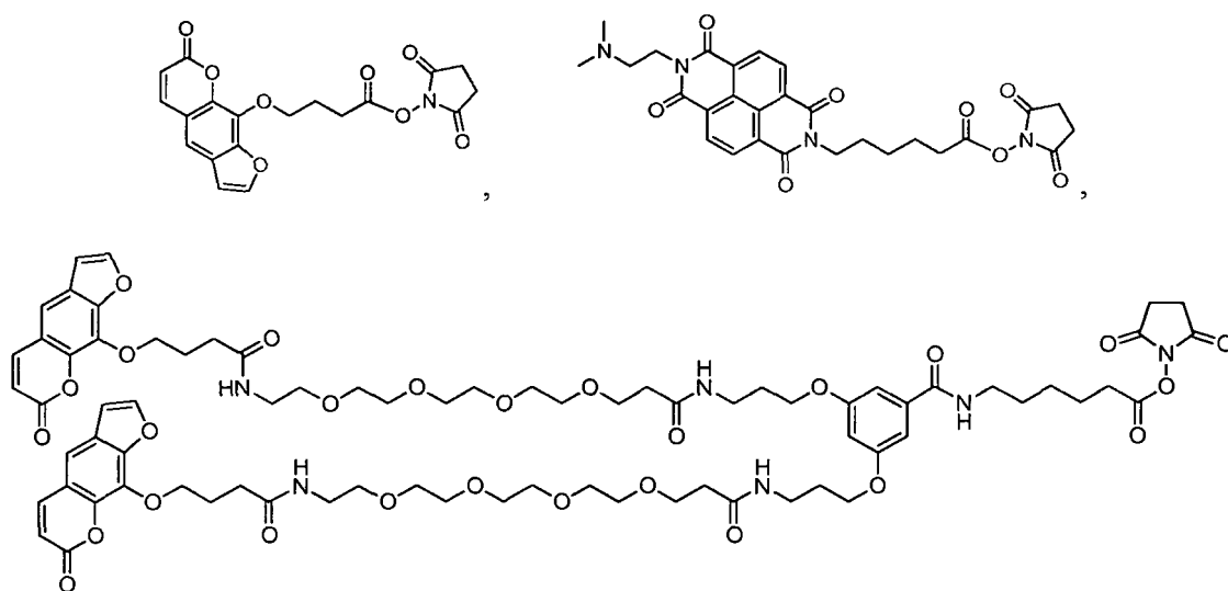
Bis-Psoralein
