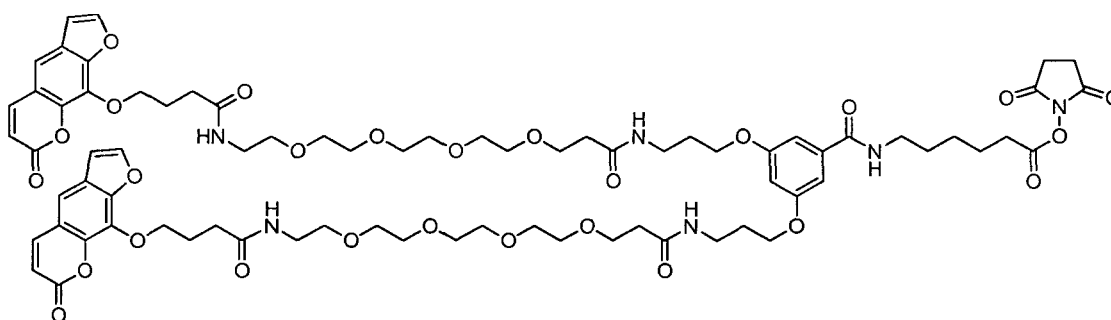
Bis -Psoralen
