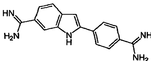
DAPI
