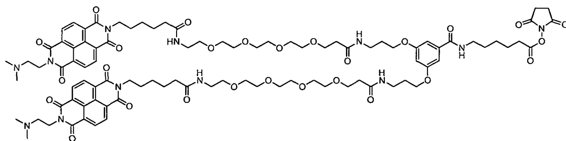
Bis-NDI-C6
