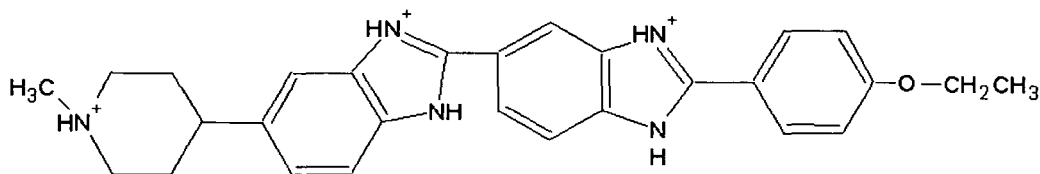
Hoechst 33342
