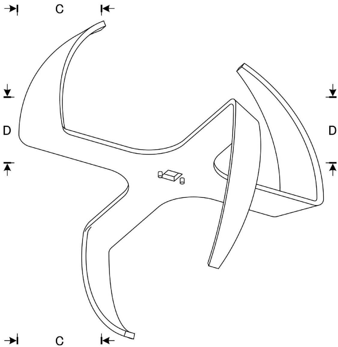
【立體圖 2】
