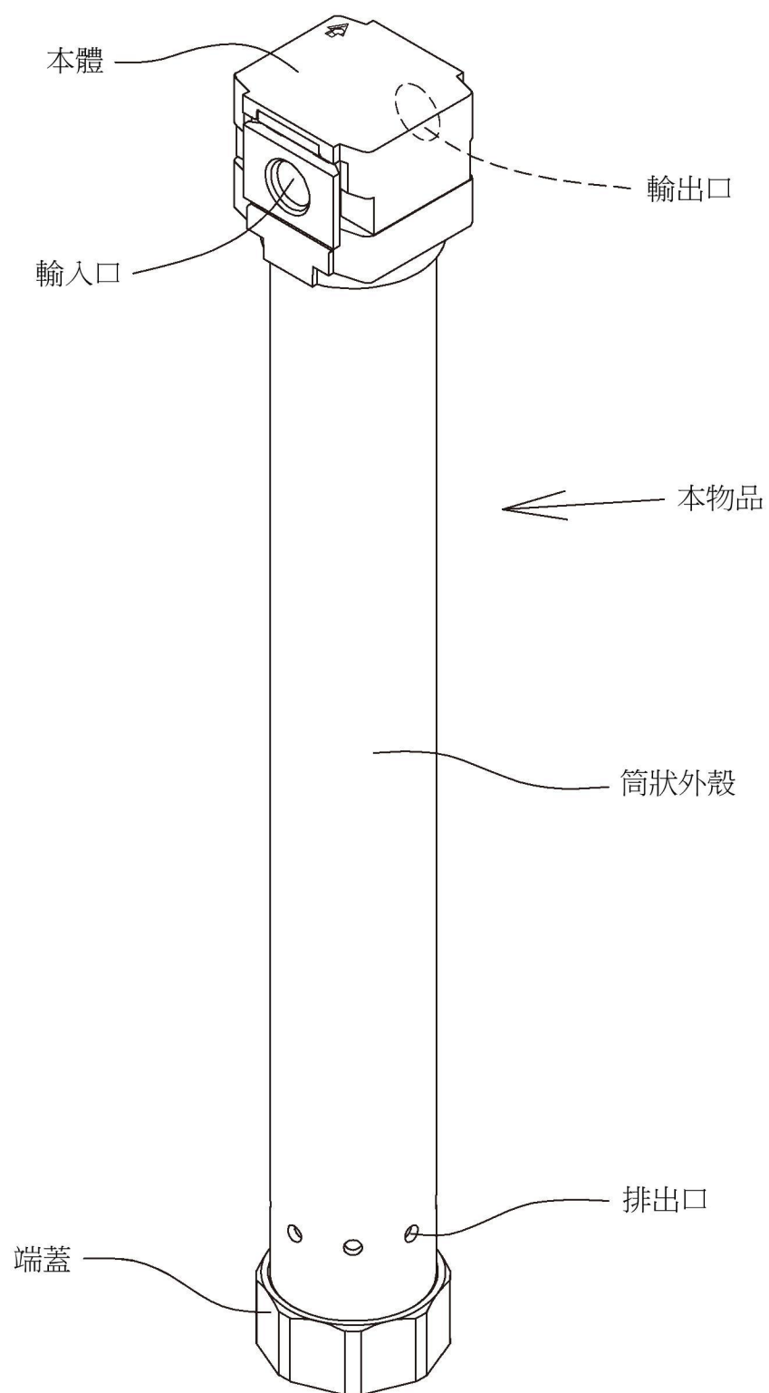
【參考圖】
