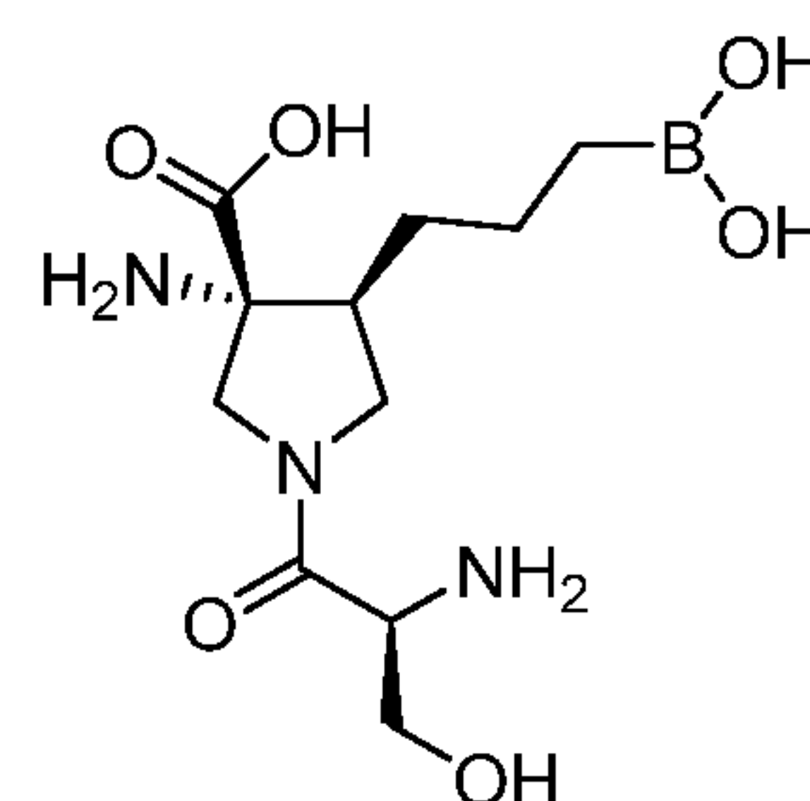
Serine AUC = 14784
