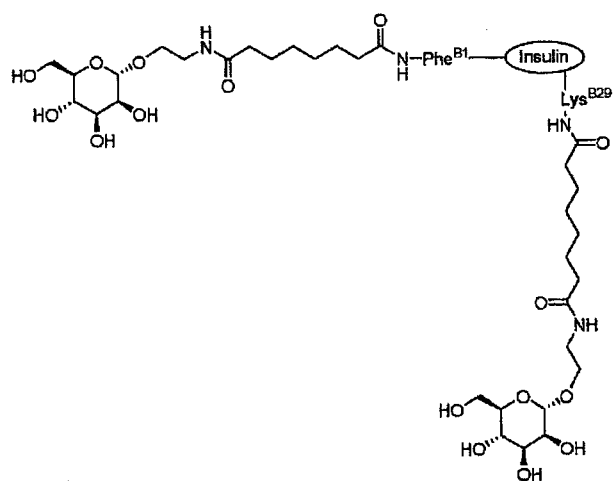
Conjugate II-7 DSS-Di-sub-AETM-2 (B1,B29)
