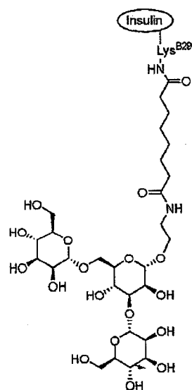
Conjugate I-10 DSS-AETM-1 (B29)
