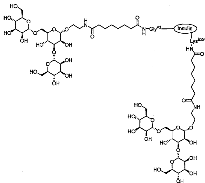
Conjugate II-3 DSS-Di-sub-AETM-1 (A1,B29)
