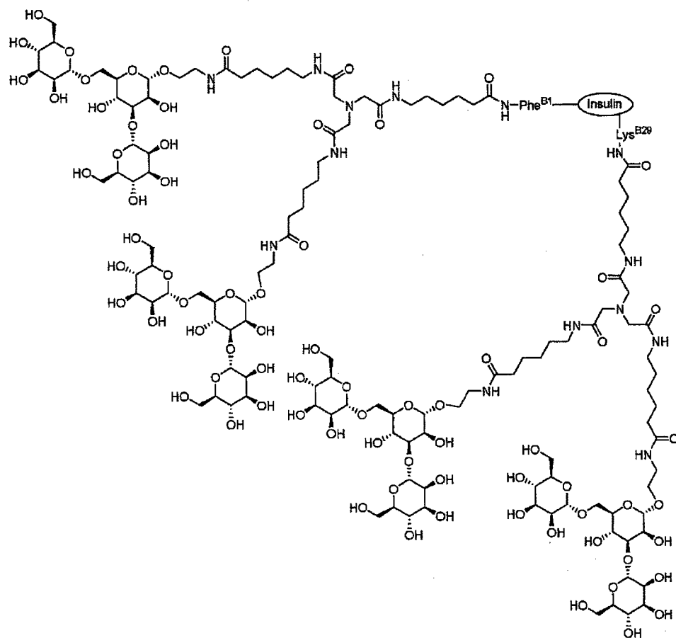
Conjugate II-6 TSAT-C6-Di-sub-AETM-2 (B1,B29)
