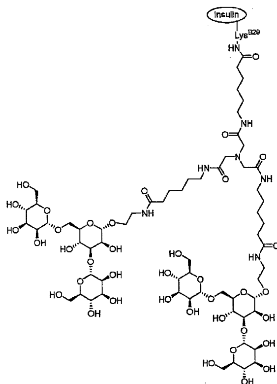
Conjugate I-6 TSAT-C6-AETM-2 (B29)
