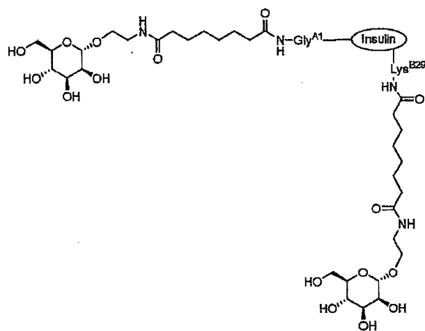
Conjugate II-4 DSS-Di-sub-AEM-1 (A1,B29)
