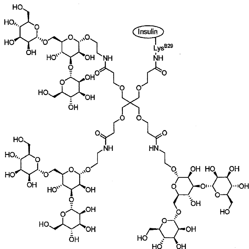
Conjugate I-11 TSPE-AETM-3 (B29)
