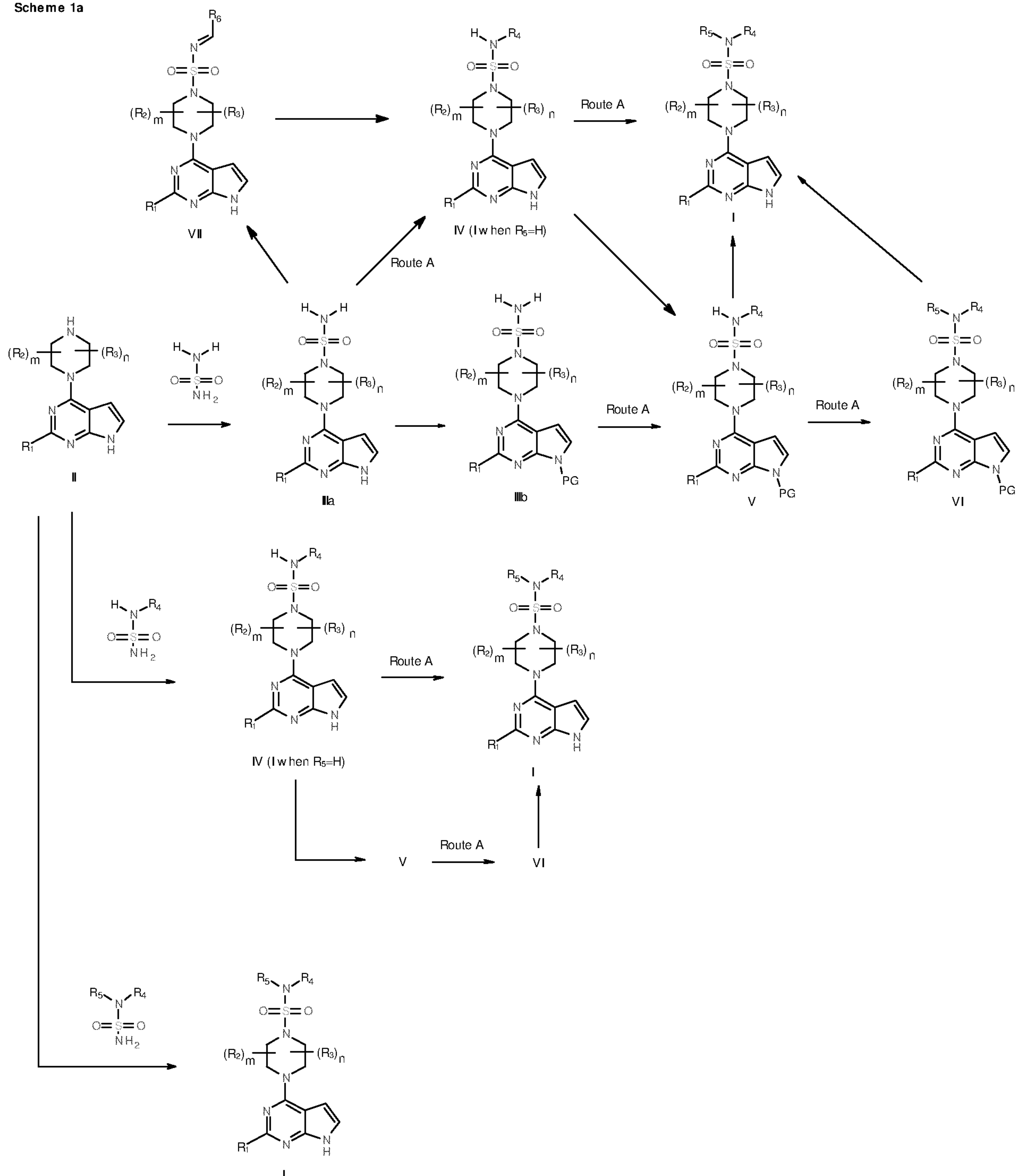
Scheme 1a
