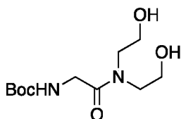
tert-butyl (2-(bis(2-hydroxyethyl)amino)-2-oxoethyl)carbamate
