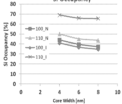
FIG. 22 Si Occupancy
