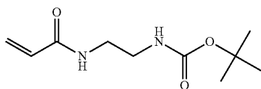
tert-butyl 2-acrylamidoethylcarbamate
