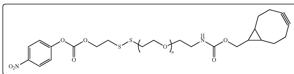
BCN—PEG2K—NPC
