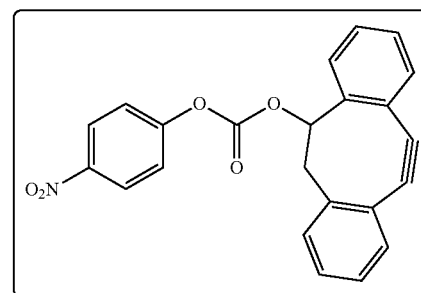
DIBO-NPC
