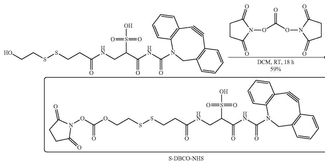
S-DBCO-NHS
