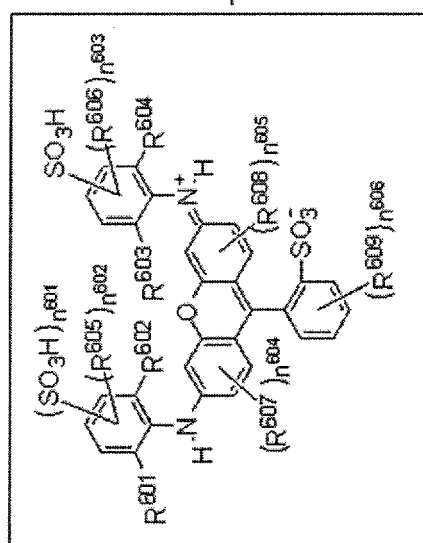
Formula (W8)
