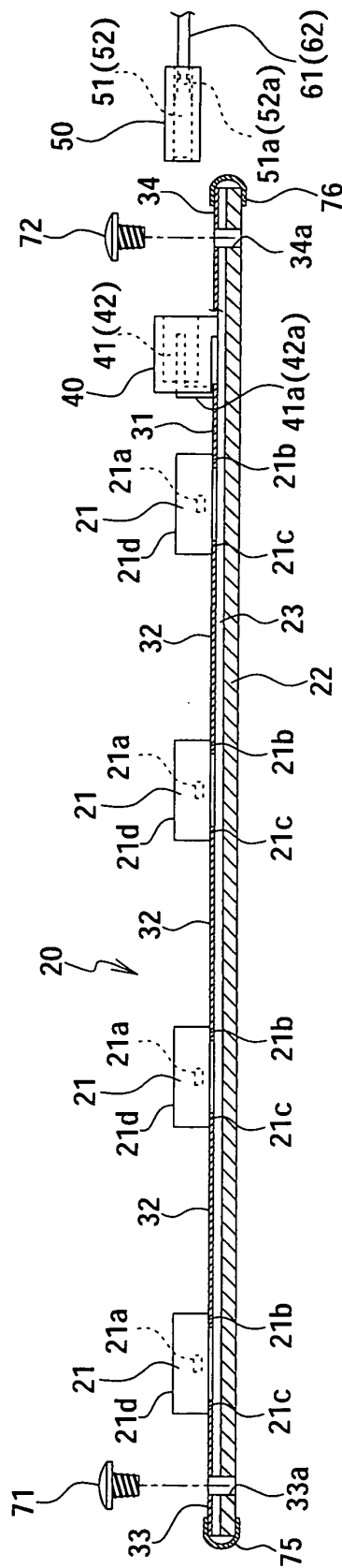
FIG. 9B
