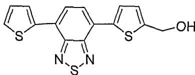
TBT-CH2OH
