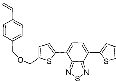
St-TBT
