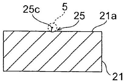
FIG. 9 (E)
