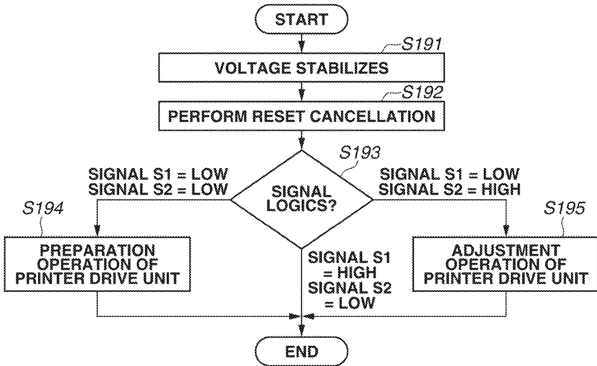
FIG.19B
