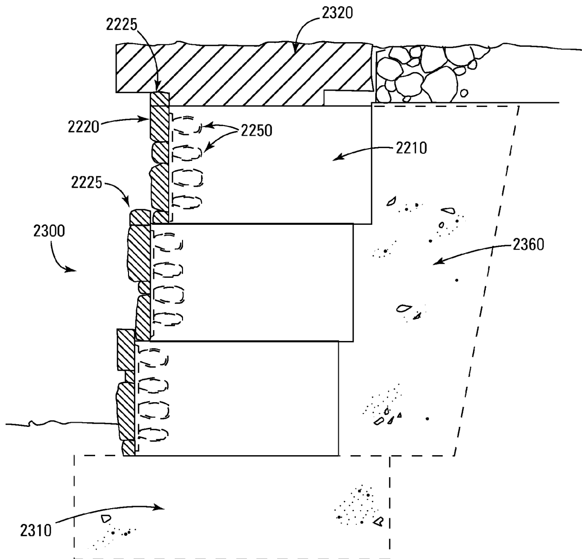
Fig. 29
