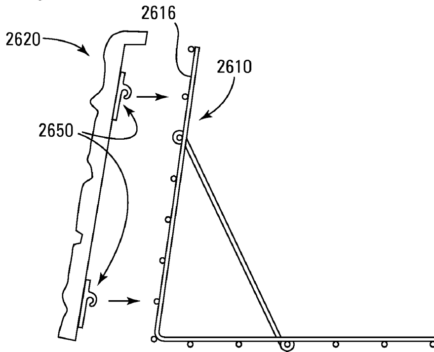
Fig. 35A
