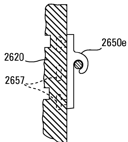
Fig. 36E
