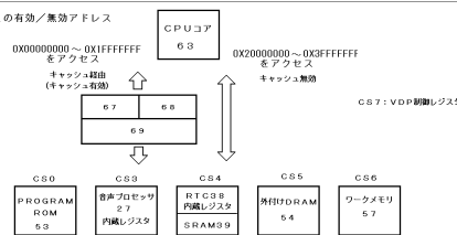
(b) キャッシュの有効/無効アドレス CRU32
