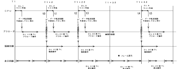
(b) 各部の動作手順を示すタイムチャート (遅延あり)
