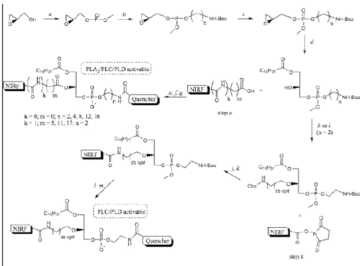
Scheme 2. Synthesis PLA2/PLC/PLD and PLC/PLD activated probes. a) MeOPCl 2 , TEA, CH 2 Cl 2 ; b) Boc-NH(CH 2 ) n OH, TEA, CH 2 Cl 2 ; c) tBuOOH, CH 2 Cl 2 ; d) C 15 H 31 CO 2 Cs, C 15 H 31 CO 2 H, DMF; e) EDC, DMAP, CH 2 Cl 2 ; f) TFA, TES, CH 2 Cl 2 ; g) Quencher-COO-NHS, Py, CH 2 Cl 2 ; h) Cbz-NH(CH 2 ) m CH 2 OC(=NH)CCl 3 , Tf-TMS; CH 2 Cl 2 ; i) Cbz-NH(CH 2 ) m CH 2 OTf, NaH, DMF; j) H 2 , Pd/C, EtOH; k) Py, CH 2 Cl 2 ; l) TFA, TES, CH 2 Cl 2 ; m) Quencher-COO-NHS, CH 2 Cl 2 , Py
