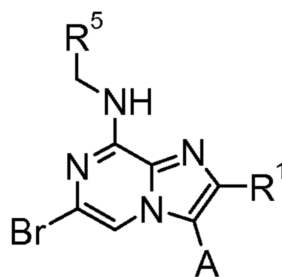
(II)
