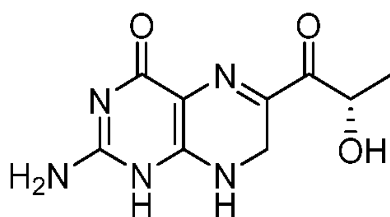
Sepiapterin
