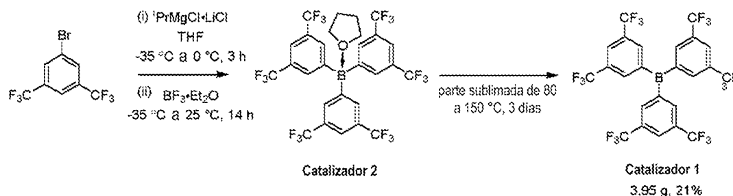
Esquema 2
