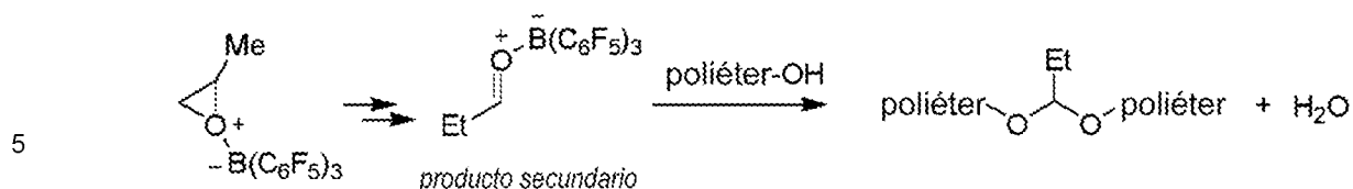
Esquema 1
