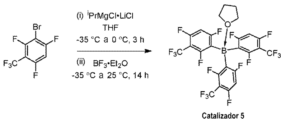
Esquema 5
