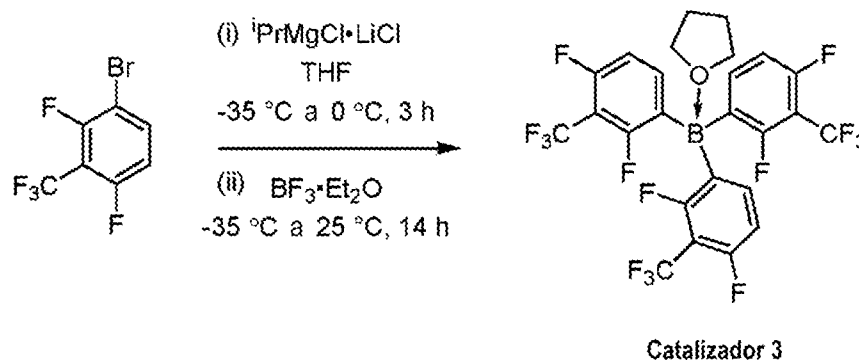
Esquema 3
