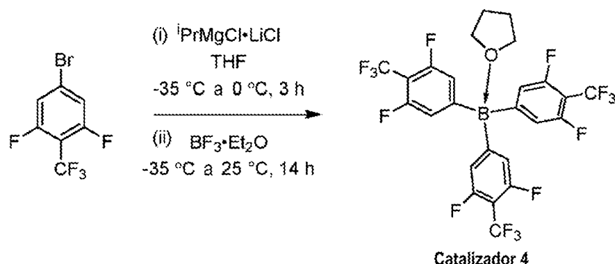
Esquema 4
