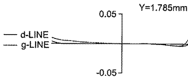
MERIDIONAL COMA (mm)
