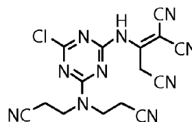
2-((4-(bis(2-cyanoethyl)amino)-6-chloro-1,3,5-triazin-2-yl) amino)prop-1-ene-1,1,3-tricarbonitrile
