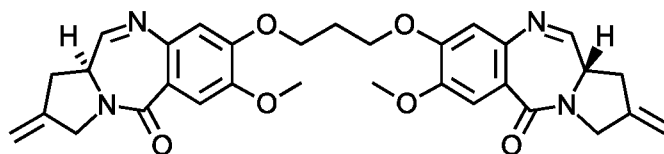
SJG-136
