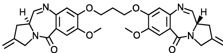
SJG-136
