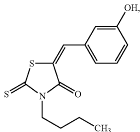
3-butyl-5-(3-hydroxybenzylidene)-2-thioxo-1,3-thiazolidin-4-one
