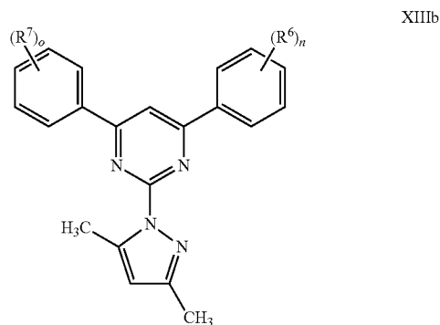
XIIIb
