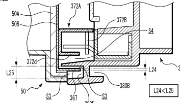
【図13-51】 開閉扉枠底部品 (特定内部進入部品と被進入部品/ドア枠所定部品と内枠所定部品)
