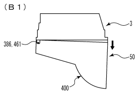
【図13-42】 開閉扉枠 [第1開状態 (開放角度: 約2度)]
