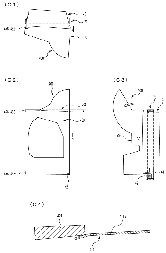
【 図 13-47 】 遊技機用枠+開閉扉枠 [第3開状態 (開放角度: 約10度)]
