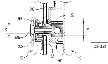
【図13-50】 球抜き通路 (特定内部進入部品と被進入部品)
