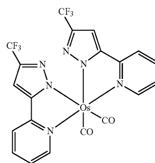
Os(fppz) 2 (CO) 2
