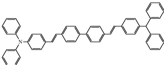
DPAVB
