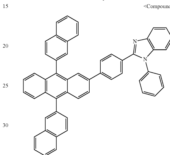
BAlq
