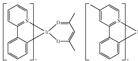
Ir(ppy) 2 (acac)
