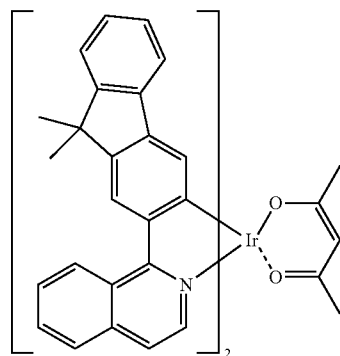
Ir(fliq) 2 (acac)
