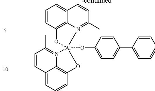
BAlq
