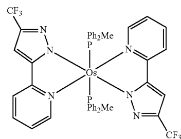
Os(fppz) 2 (PPh 2 Me) 2
