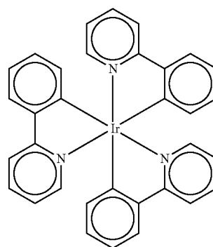
Ir(ppy) 3
