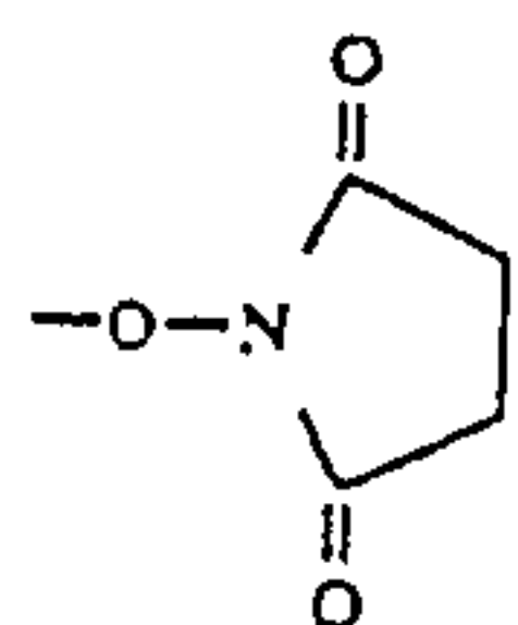
Oxysuccinimide
