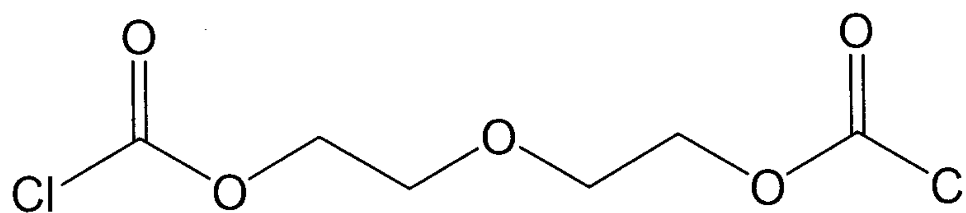
diethylene glycol bischloroformate.
