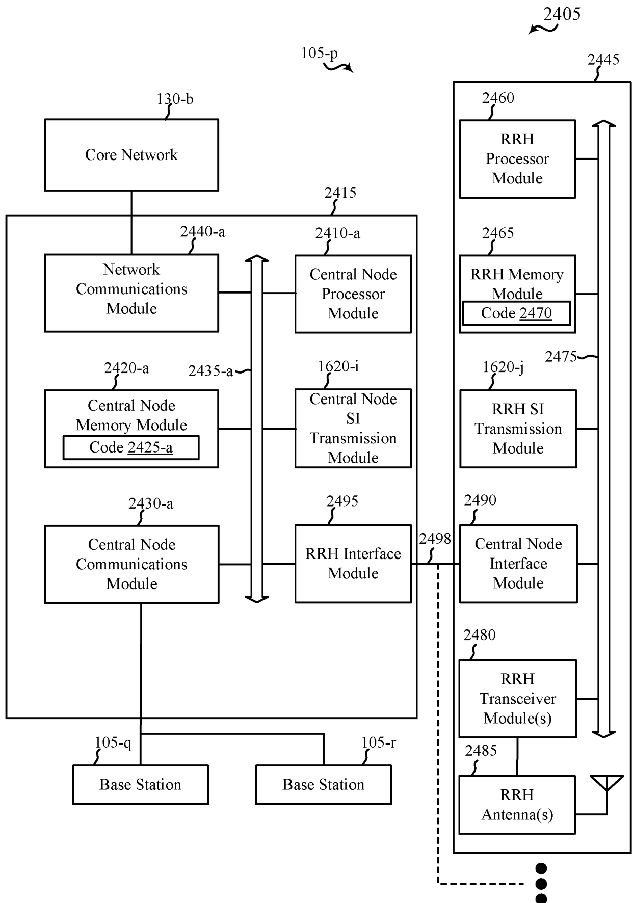
FIG. 24B
