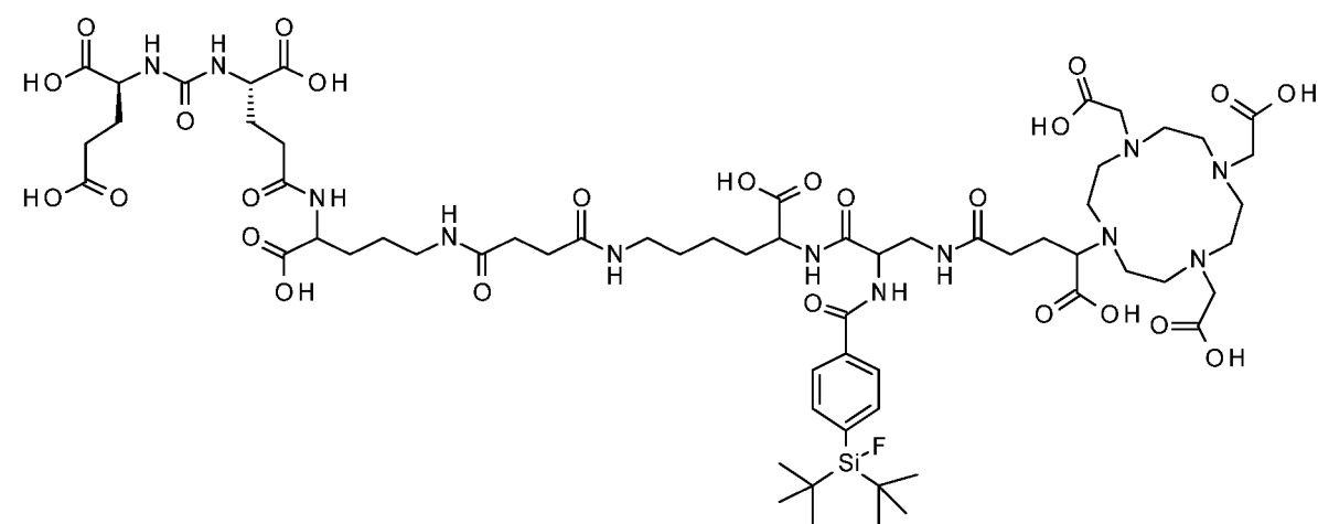
PSMA-SIFA4 (8)
