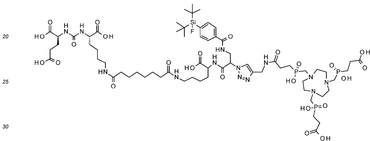
PSMA-SIFA2 (6)
