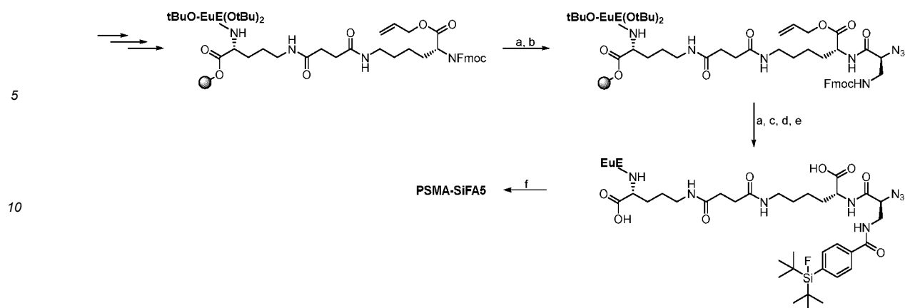
Scheme 5: Synthesis of PSMA-SIFA5: a) 20% piperidine, (DMF); b) N 3 -L-Dap(Fmoc)-OH, HOBT, TBTU, DIPEA, (DMF); c) SIFA-BA, HOBT, TBTU, DIPEA (DMF); d) TIPS, Pd(PPh 3 ) 4 , (DCM); e) TFA; f) propargyl-TRAP, Cu(OAc) 2 ·H 2 O, sodium ascorbate (tBuOH, H 2 O).
