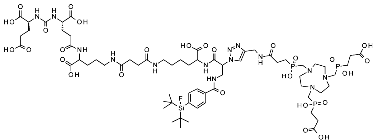
PSMA-SIFA5 (9)
