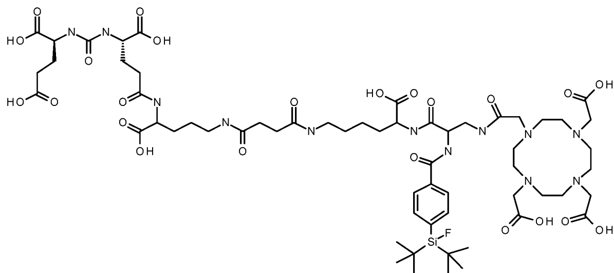
PSMA-SIFA 11
