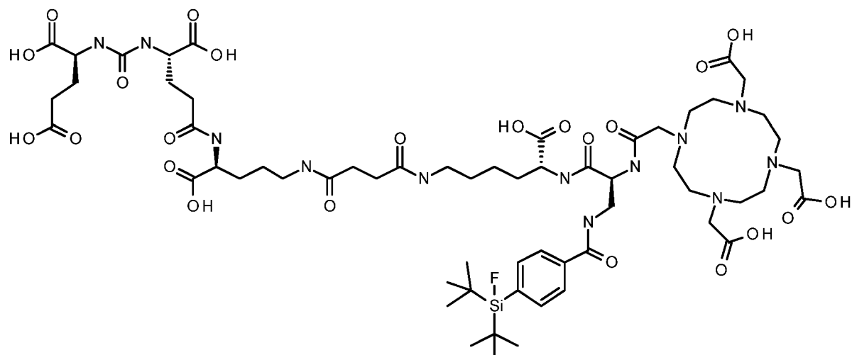
PSMA-SIFA 11
