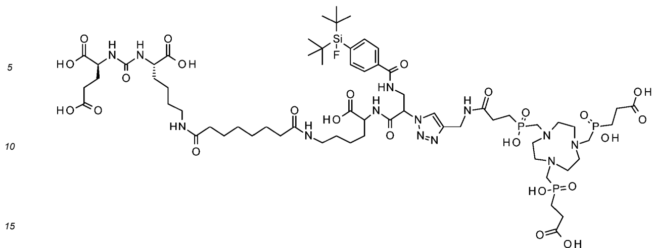
PSMA-SIFA3 (7)
