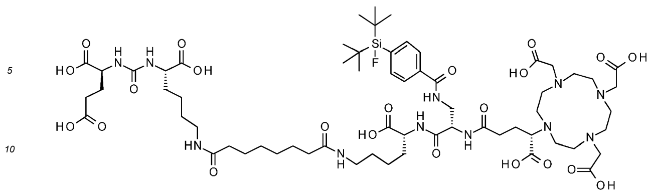
PSMA-SIFA2 (6)
