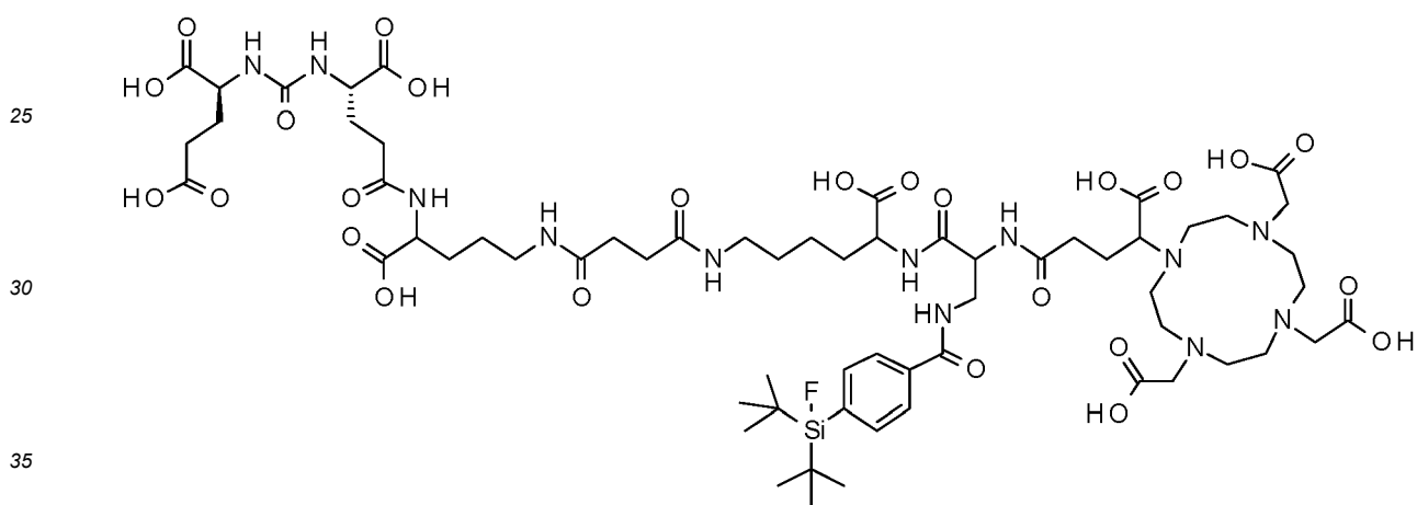
PSMA-SIFA4 (8)
