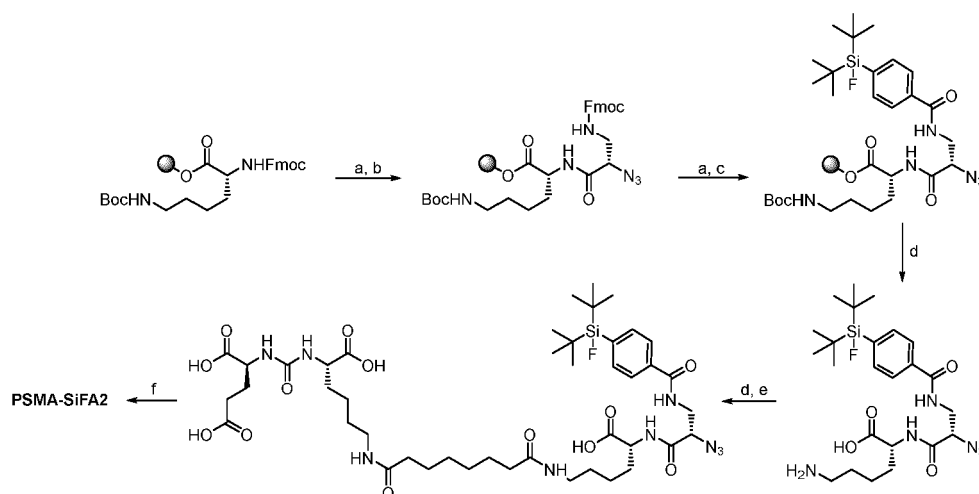
Scheme 2: Synthesis of PSMA-SIFA2: a) 20% piperidine (DMF); b) N 3 -L-Dap(Fmoc)-OH, HATU, HOAt, DIPEA (DMF); c) SIFA-BA, HOBt, TBTU, DIPEA (DMF); d) TFA; e) PfpO-Sub-(tBuO)-KuE(OtBu) 2 , TEA, (DMF); f) propargyl-TRAP, Cu(OAc) 2 ·H 2 O, sodium ascorbate (tBuOH, H 2 O).
