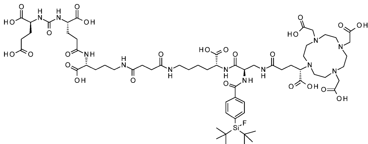
PSMA-SIFA5 (9)
