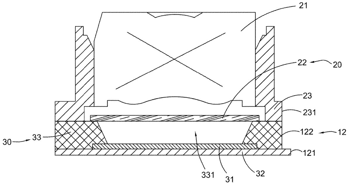
A-A Fig.3
