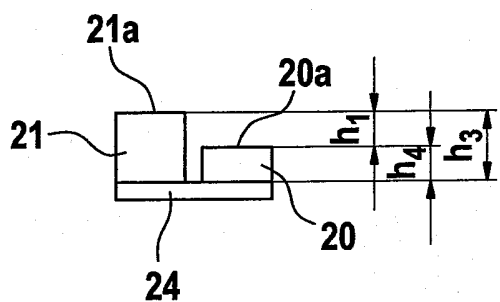
Fig.4e Schnitt A-A
