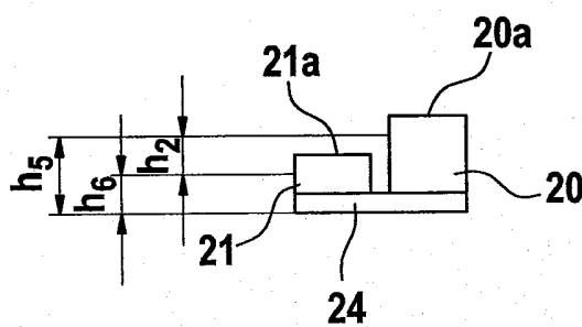
Fig.4g Schnitt C-C
