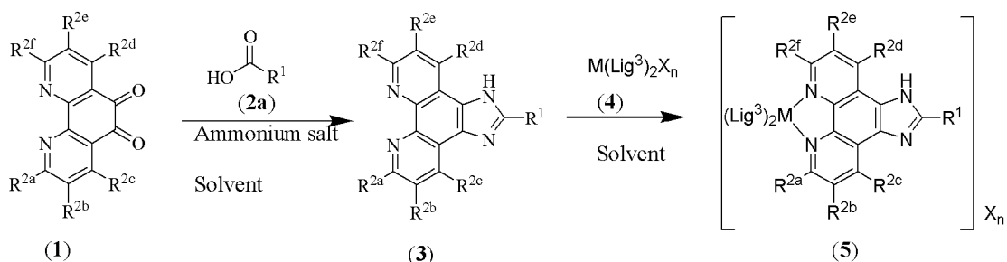
Scheme 1a
