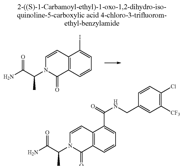
a. (S)-2-(1-Amino-1-oxopropan-2-yl)-N-(4-chloro-3-(trifluoromethyl)benzyl)-1-oxo-1,2-dihydroisoquinoline-5-carboxamide
