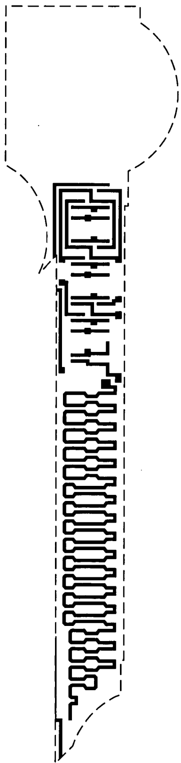
Poly mask
