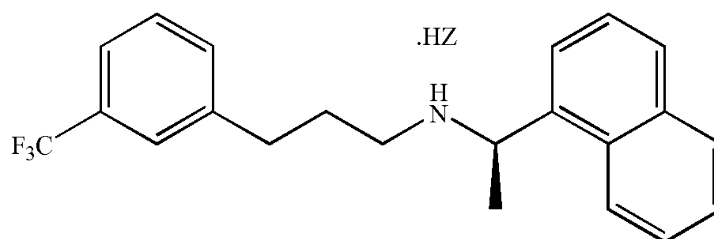
(Ia)
