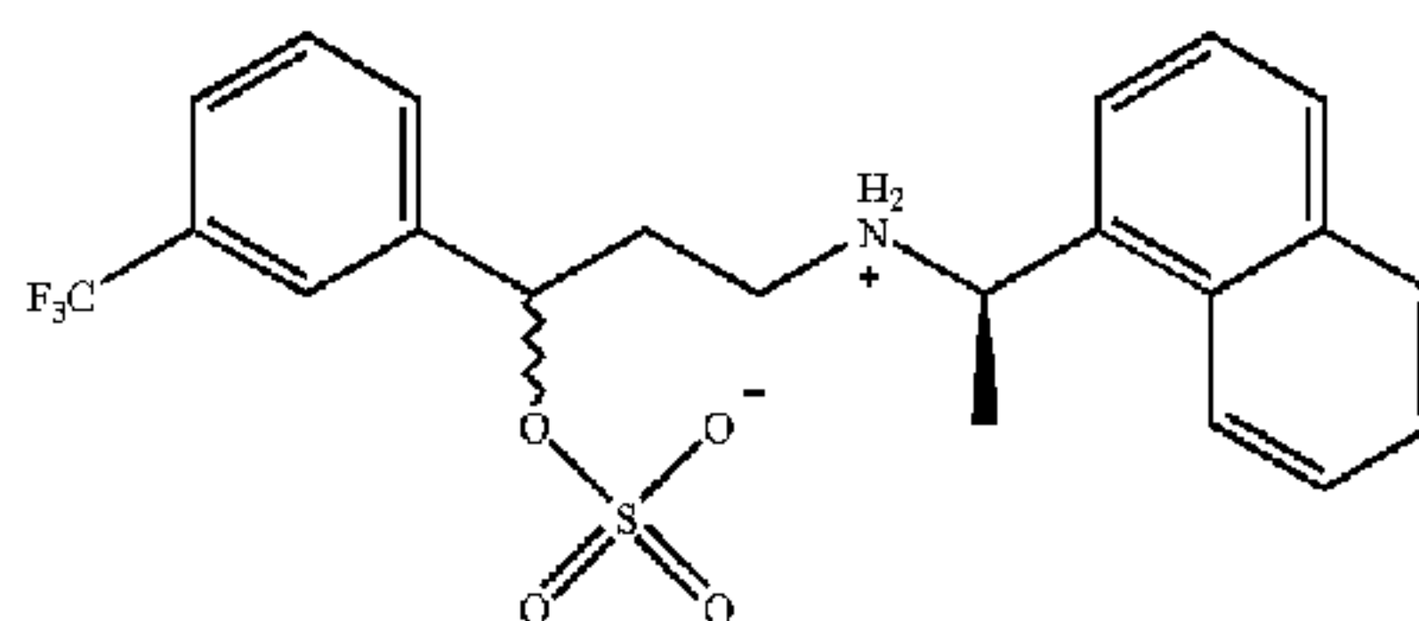
(VIII)
