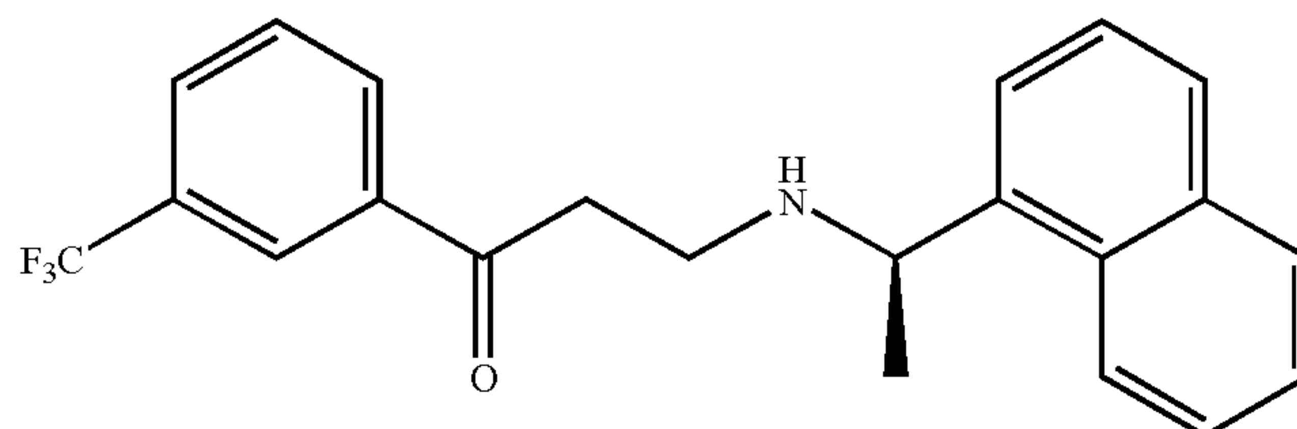
(V)
