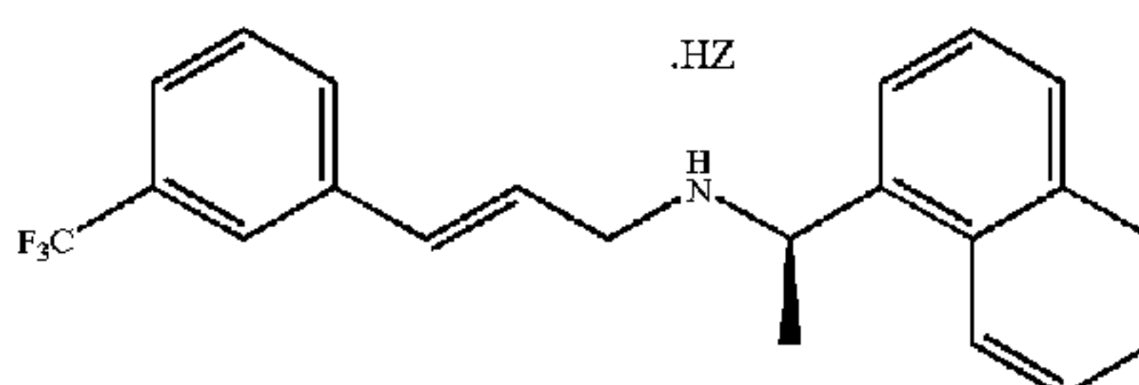
(VII)
