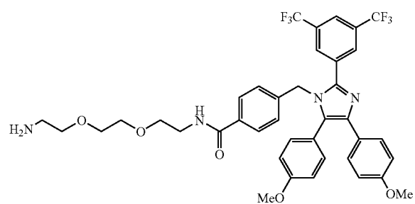
Apoptozole 2
