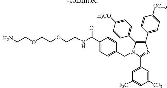
Apoptozole 2
