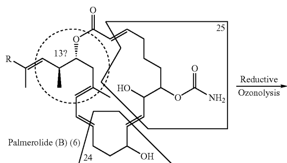
Scheme 4. Ozonolysis of palmerolide B (6).
