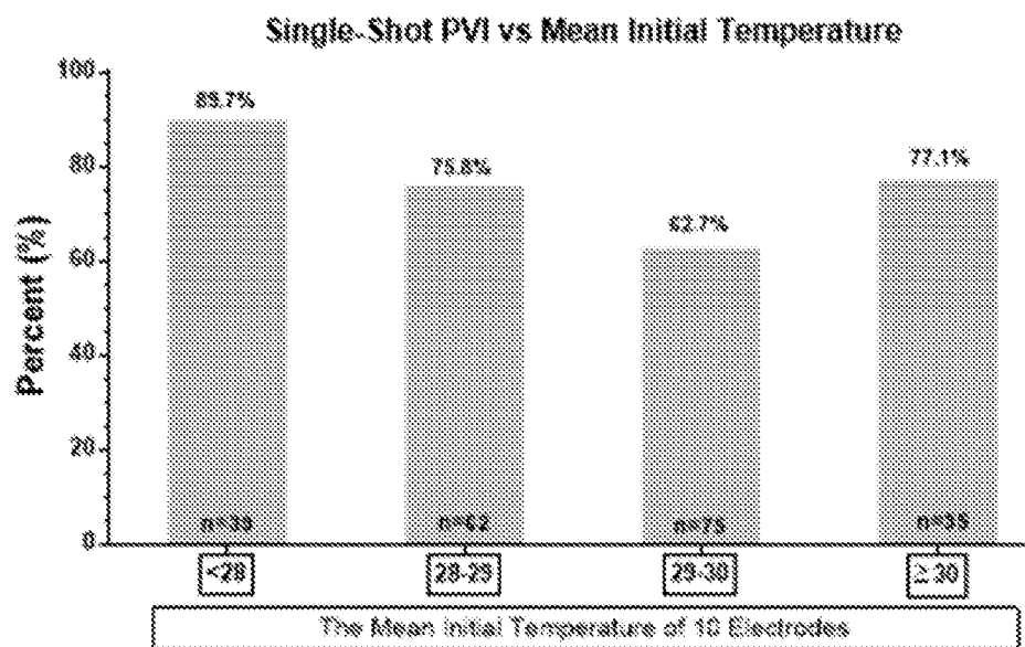
Fig. 75A
