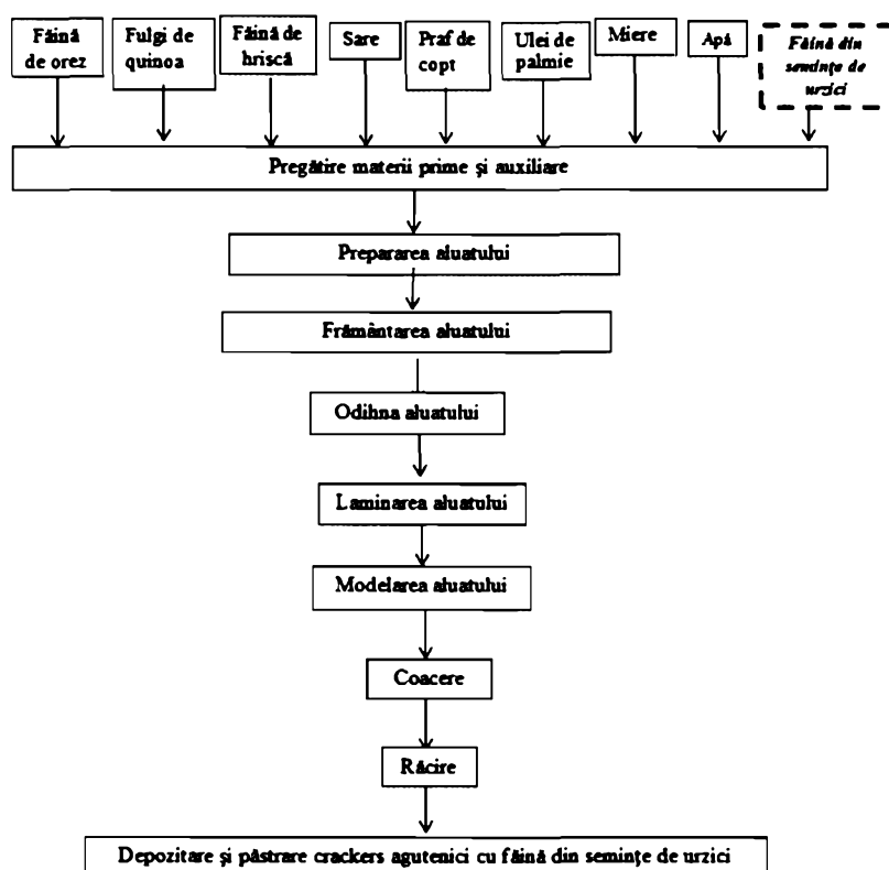
Figura 4. Schema tehnologică de fabricare a crackerslor din făină de orez, quinoa și hrișcă cu adaos de făină din semințe de urzici
