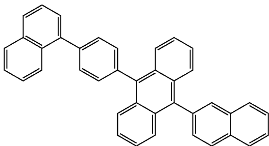
Emitter 1:
