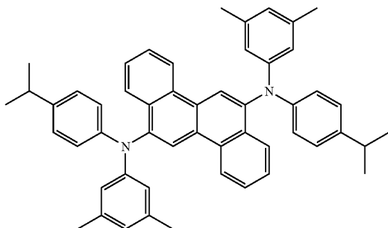
Emitter 1:
