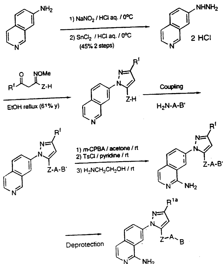
SCHEME 2a
