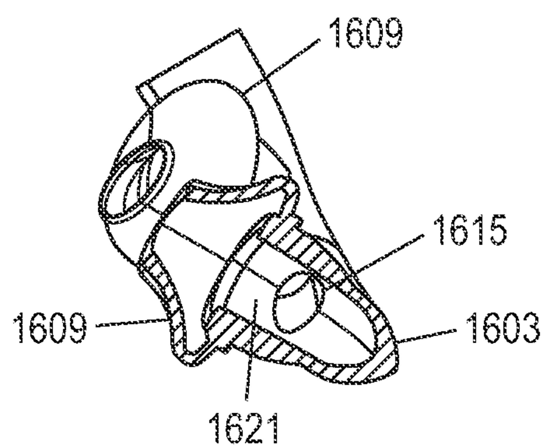
FIG. 19C SECTION G-G
