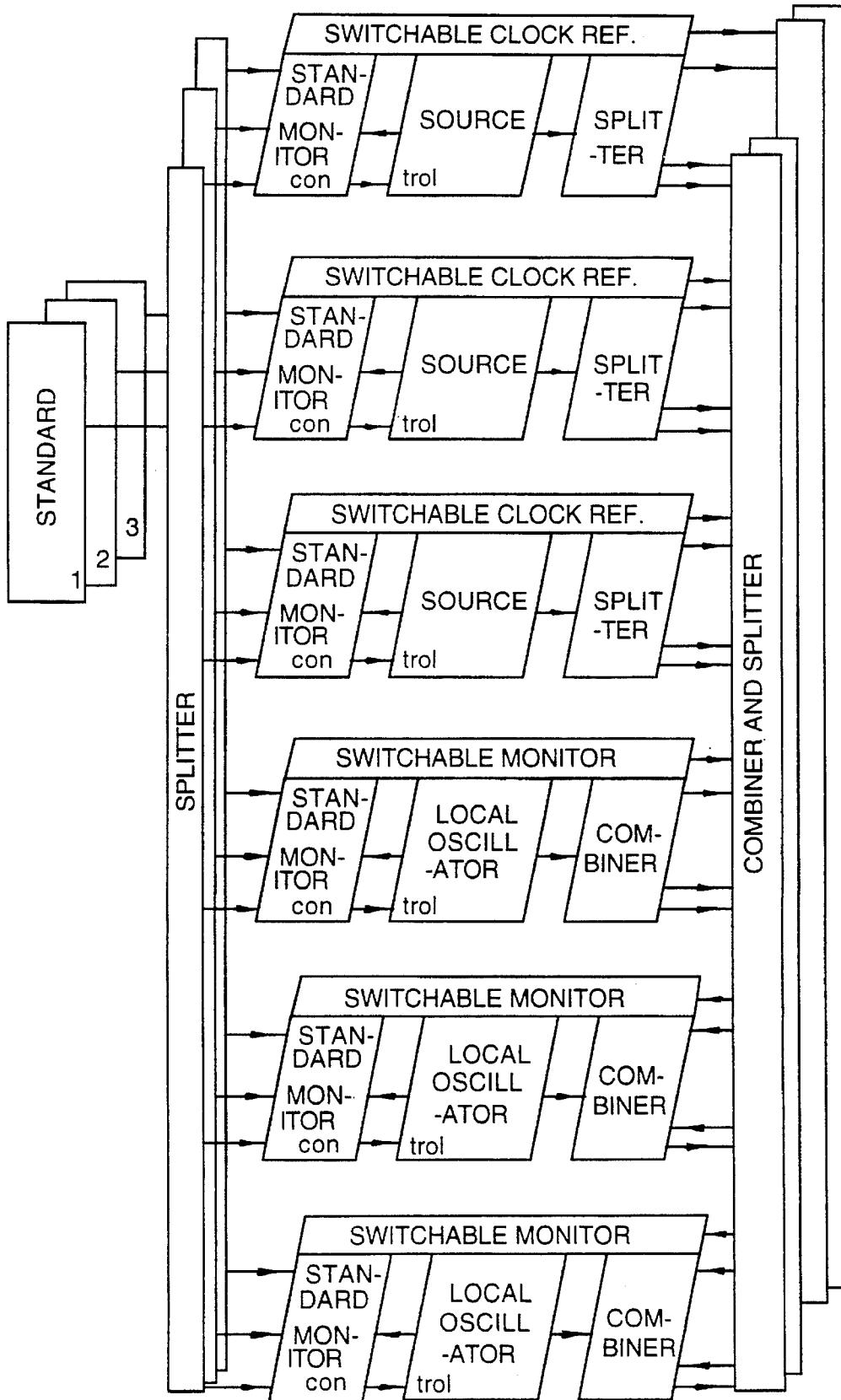
CLOCK STABILISATION FIG. 3J
