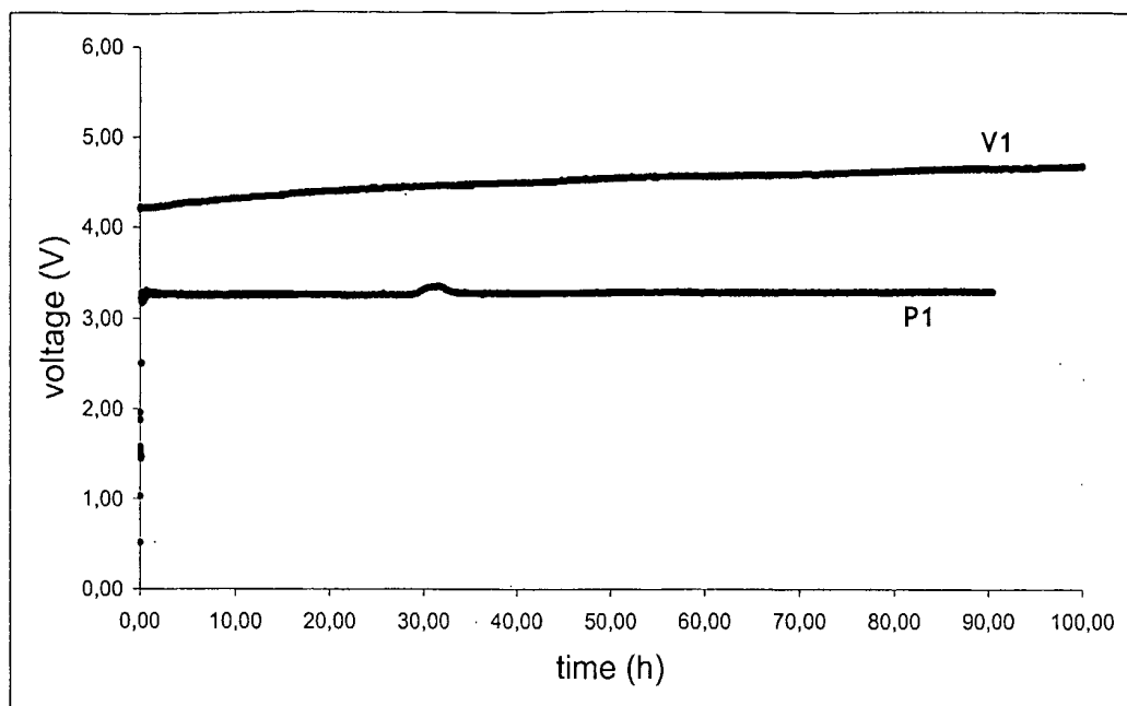
Figur 1: Spannung in Abhängigkeit der Zeit bei konstanter Stromdichte
