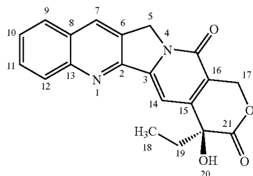
camptothecin
