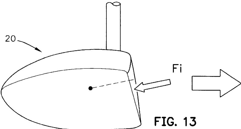
De-lofting Force
