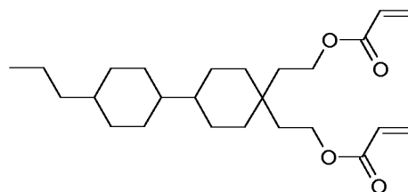
RM-19
