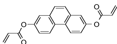
RM-7
