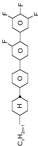
PYP-n-F
