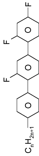
LYLI-n-m
