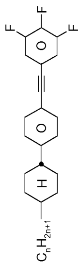
CCOC-n-m
