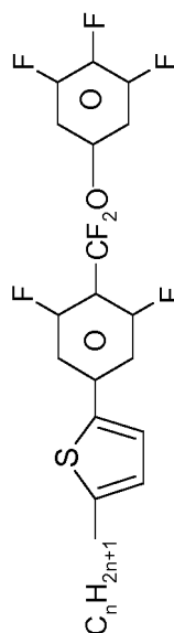
SUQU-n-F
