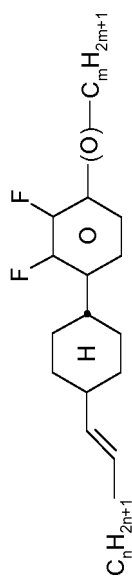
CY-nV-(O)m
