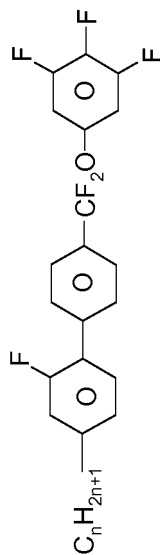
PGUQU-n-F
